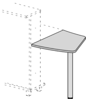
Стол приставной 31R004 768*817*735 мм
